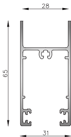
MT-6501 Cabezal y zócalo corrediza 90° Peso estimado: 0.848 Kg/m Largo STD: 6200 mm
