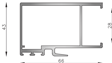
MT-6504 Parante central de hoja 90° Peso estimado: 1.204 Kg/m Largo STD: 6200 mm
