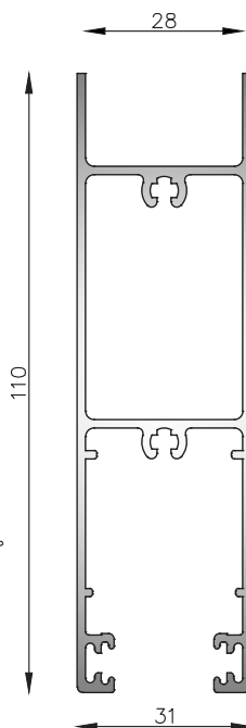
MT-6502 Zócalo alto corrediza 90° Peso estimado: 1.396 Kg/m Largo STD: 6200 mm
