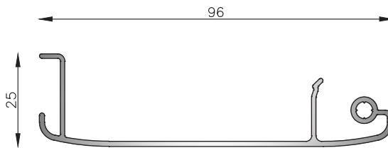
MT-0245 Tapa cinta Peso estimado: 0.623 Kg/m Largo STD: 6150 mm
