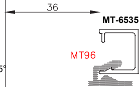
MT-6535 Contravidrio recto interior 15mm a 45° Peso estimado: 0.166 Kg/m Largo STD: 6030 mm
