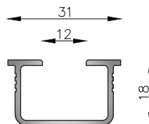
MT-6508 Adaptador VS 90° Peso estimado: 0.286 Kg/m Largo STD: 6200 mm
