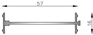
MT-0401 Acople a 180°, módulo de 60mm Peso estimado: 0.343 Kg/m Largo STD: 6200 mm
