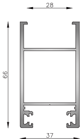
MT-6503 Parante lateral de hoja 90° Peso estimado: 1.226 Kg/m Largo STD: 6200 mm
