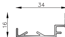
MT-0415 Tapa junta recto Peso estimado: 0.200 Kg/m Largo STD: 6150 mm
