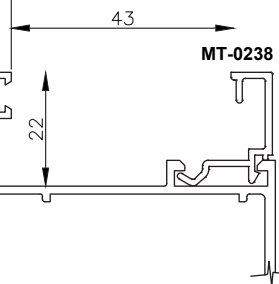
MT-0238 Contravidrio recto interior 8mm Peso estimado: 0.183 Kg/m Largo STD: 6030 mm
