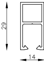
MT-6505 Tope mosquitero 90° Peso estimado: 0.316 Kg/m Largo STD: 6200 mm
