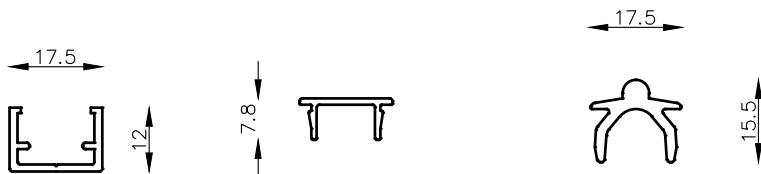
MT-6545 Tapa parante lateral Área: 34 mm 2 Peso: 0.097 Kg/m.-
