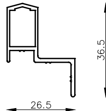
MT-6554 Perfil guía de mosquitero Área: 117 mm 2 Peso: 0.316 Kg/m.-
