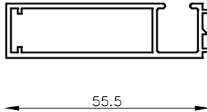
MT-6517 Premarco Área: 197 mm 2 Peso: 0.532 Kg/m.-
