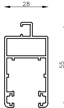
MT-6151 Hoja Mosquitero Super Reforzado Área: 271 mm 2 Peso: 0.732 Kg/m.-
