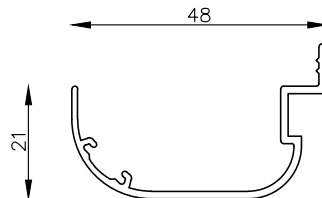
MT-3202 Tapa junta curvo Peso estimado: 0.348 Kg/m Largo STD: 6200 mm
