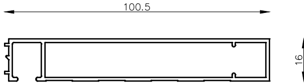
MT-6516 Premarco 3 Guías Área: 321 mm 2 Peso: 0.867 Kg/m.-
