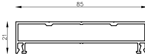
MT-6542 Marco Lateral Área: 320 mm 2 Peso: 0.864 Kg/m.-
