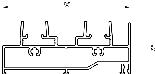
MT-6539 Marco Umbral Área: 517 mm 2 Peso: 1.396 Kg/m.-
