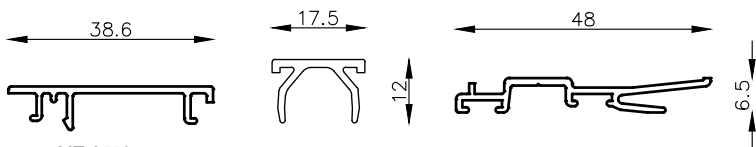
MT-6555 Guía para paño fijo Área: 59 mm 2 Peso: 0.159 Kg/m
