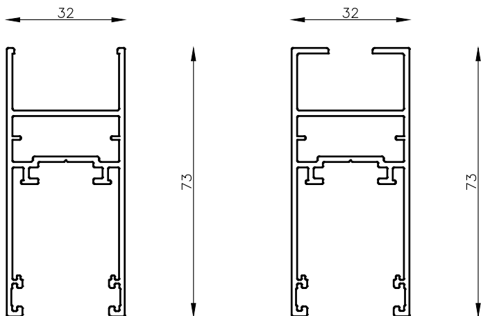
MT-6548 Hoja perimetral DVH Área: 357 mm 2 Peso: 0.963 Kg/m.- Jx: 6,3978 cm 4 Wx: 3,9986 cm 3
