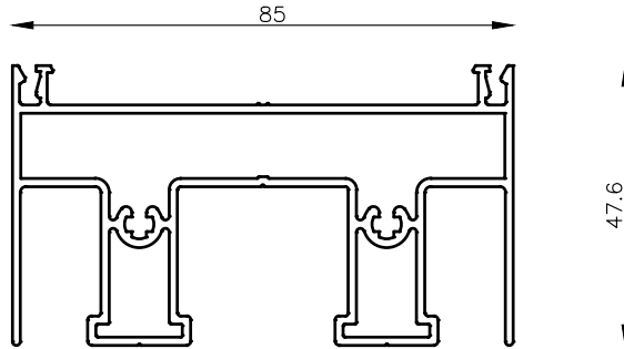
MT-6546 Marco Dintel Área: 611 mm 2 Peso: 1.649 Kg/m.-
