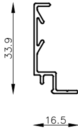
MT-0415 Tapa junta Peso: 0.200 Kg/m.-
